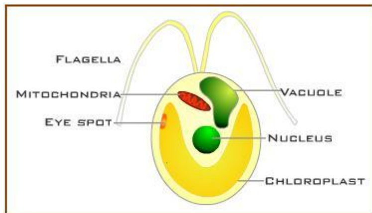
Chlamydomonas
