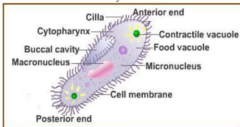
Paramecium
